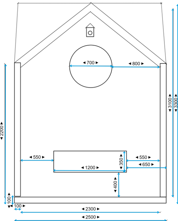
TYŁ BACK
