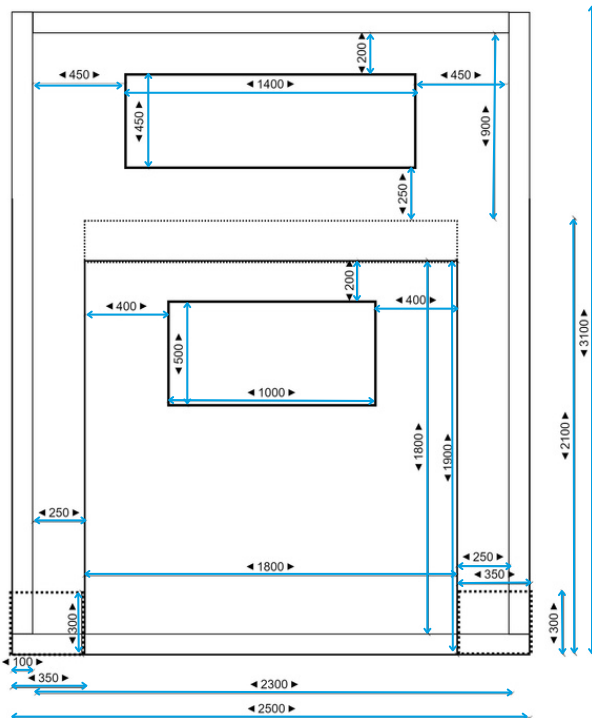
PRZÓD FRONT
