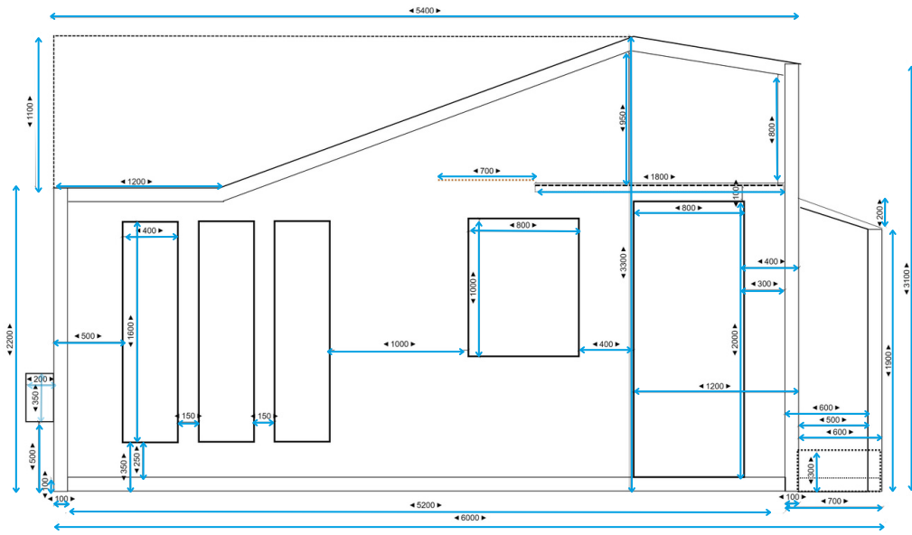
PRAWA STRONA RIGHT SIDE
