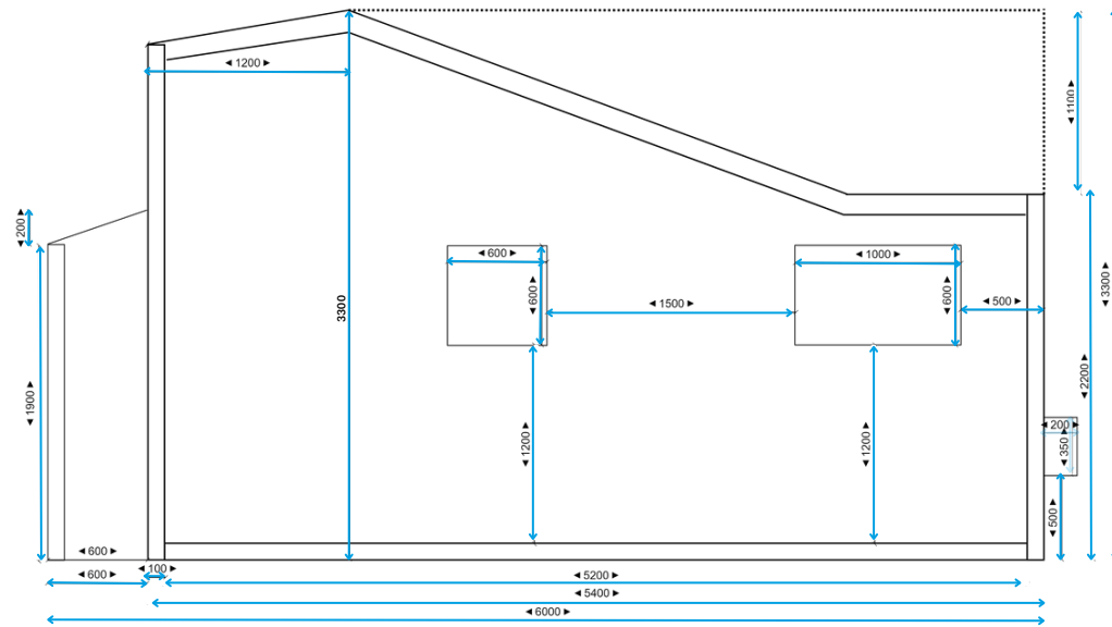
LEWA STRONA LEFT SIDE
